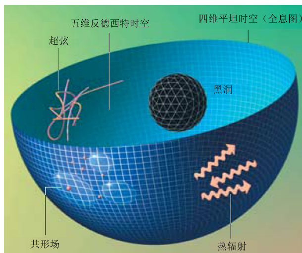
图3 AdS空间的全息图
